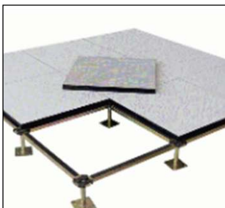
PANEL ANTIESTÁTICO / CALCIUM FS800 - FS1250
