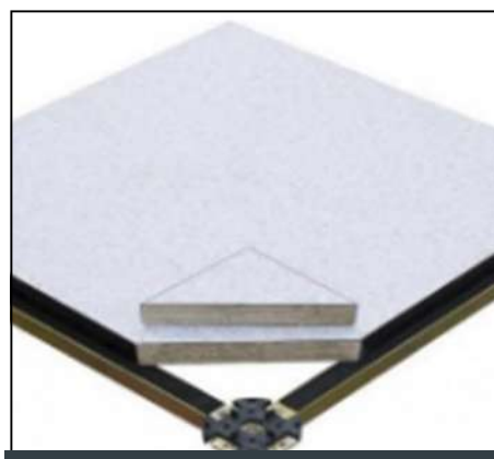
PANEL ANTIESTÁTICO / WOODCORE FS662 - FS1250
